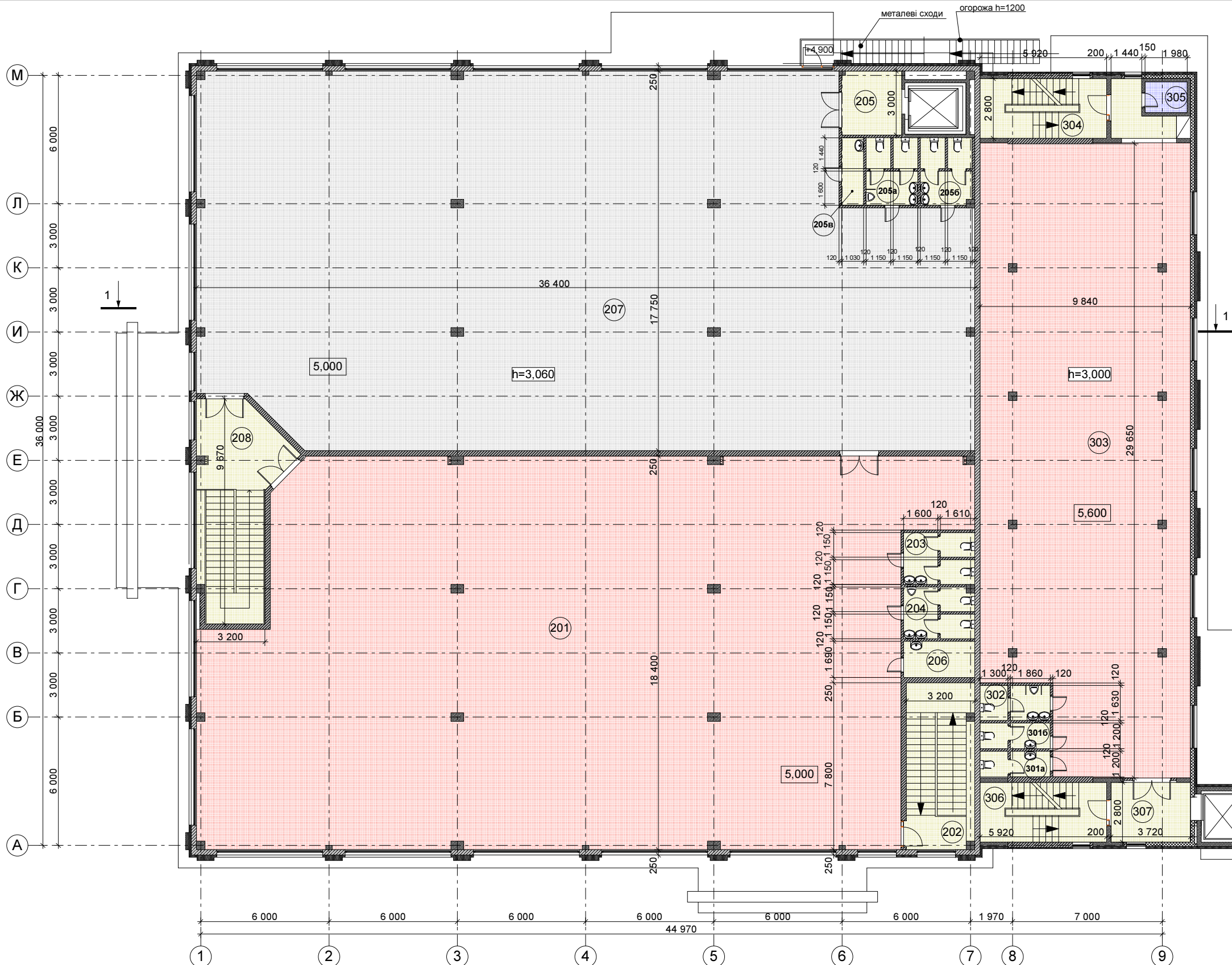
План на позн. +5,000 (2 поверх); +5,600 (3 поверх)
