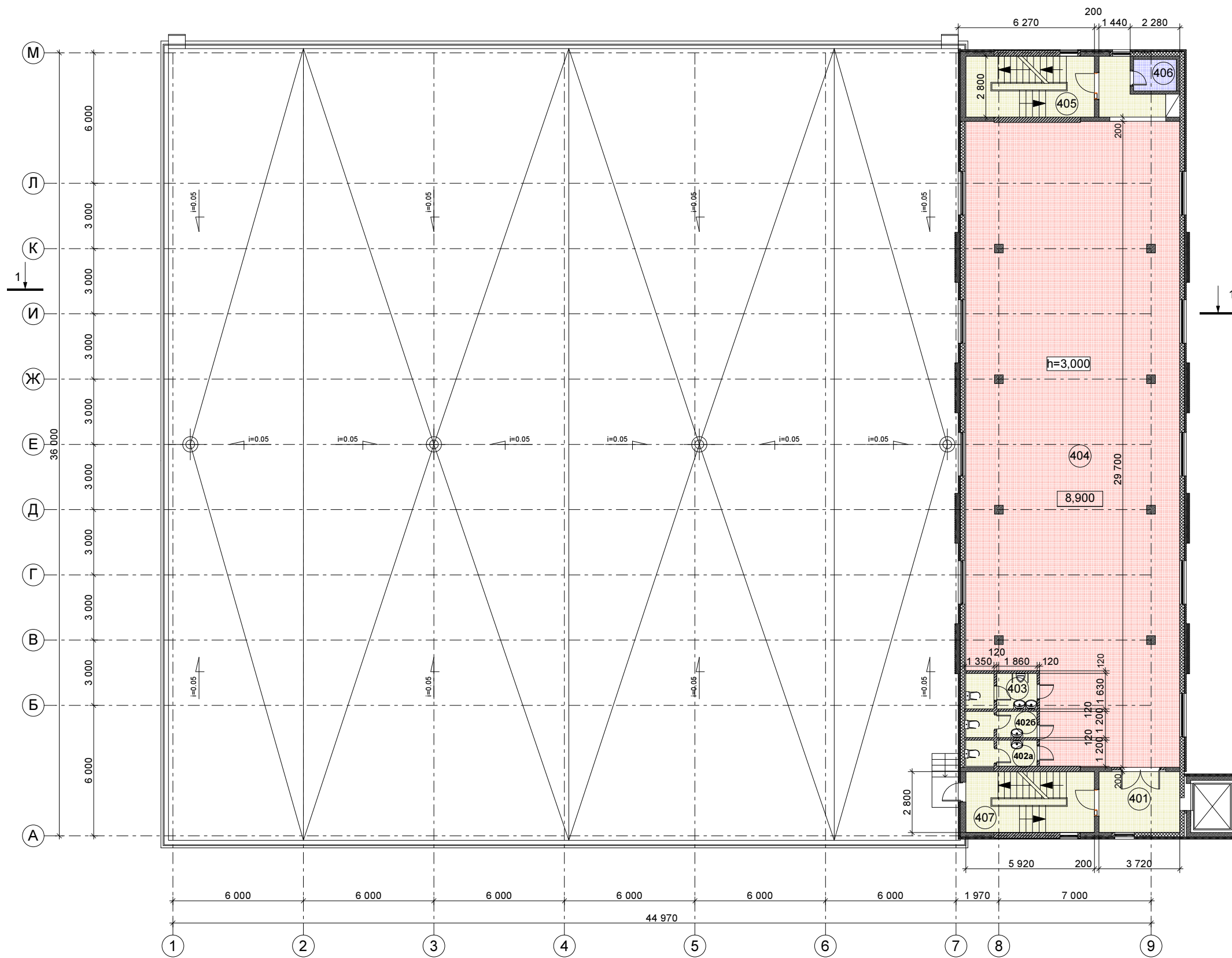
План на позн. +8,900 (4 поверх)
